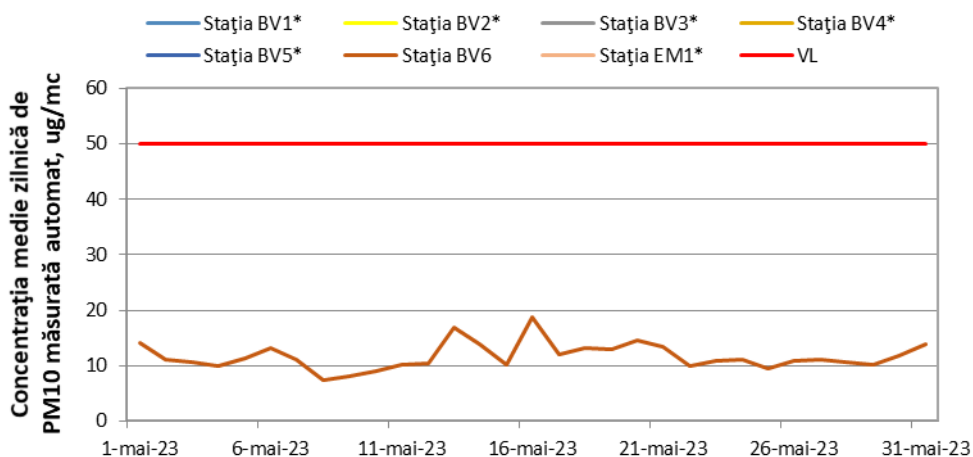
Figura 1.1.2.4.3. Evoluția mediilor zilnice de PM 10, metoda automată, în luna mai
