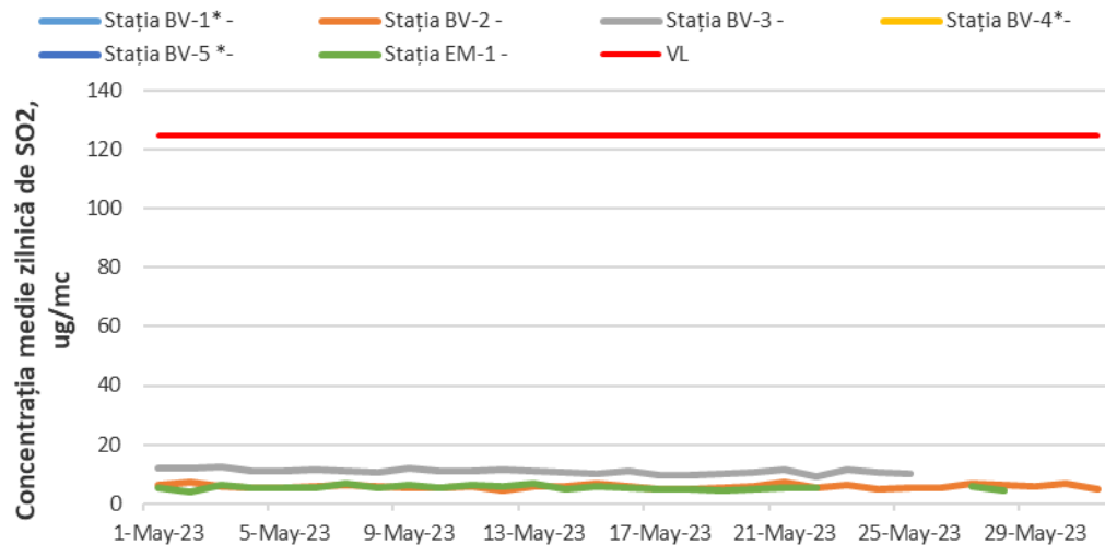
Figura 1.1.2.1.1. Evoluția mediilor zilnice de SO 2 în luna mai
