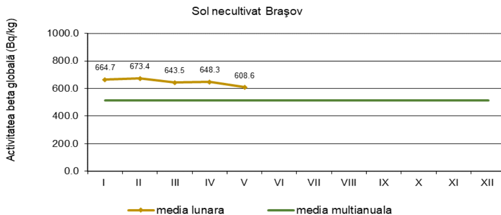
Fig. 1.2.8. Activitatea beta globală la 5 zile a solului necultivat
