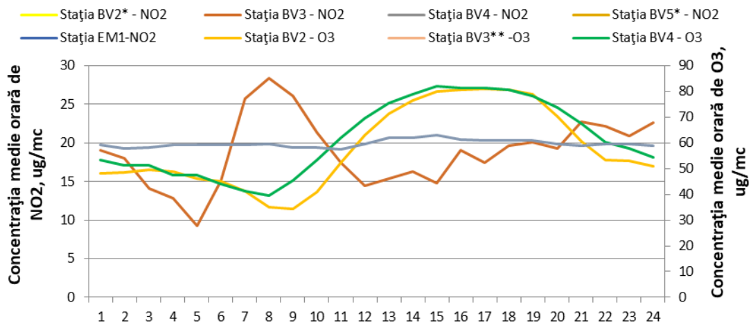
Figura 1.1.2.3.4. Ciclul zilnic al O 3 și NO 2
