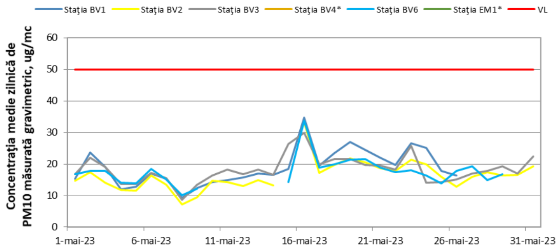
Figura 1.1.2.4.1. Evoluția mediilor zilnice de PM 10 (gravimetric) în luna mai
