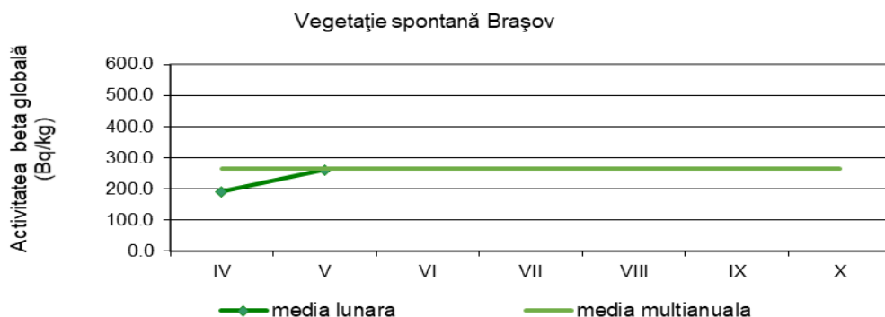
Fig. 1.2.9. Activitatea beta globală la 5 zile a solului necultivat
