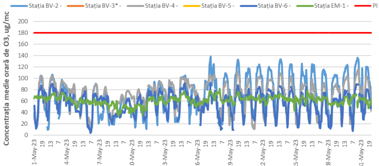
*captura de date valide în luna aprilie a fost de 0% la stația BV3 și la stația BV5 din motive tehnice Figura 1.1.2.3.1. Evoluția concentrațiilor medii orare de \text{O}_3 în luna mai
