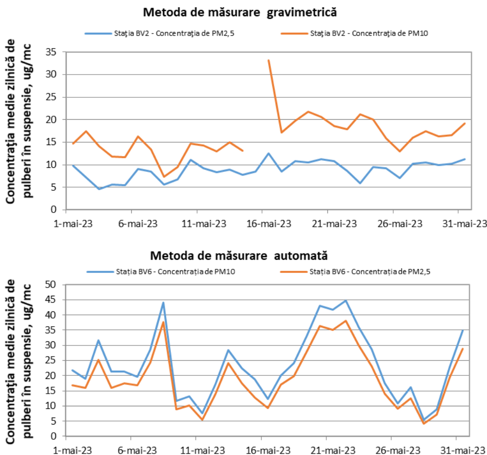
Figura 1.1.2.4.4 Evoluția mediilor zilnice de PM 2,5 și PM10 în luna mai
