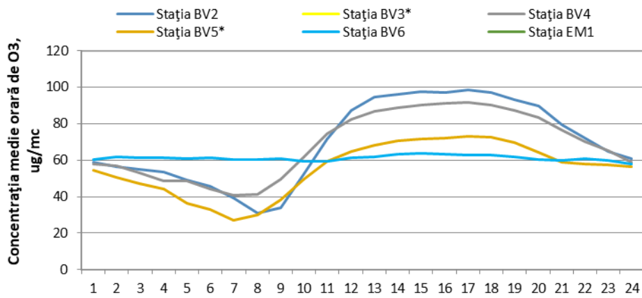
Figura 1.1.2.3.3. Ciclul zilnic al ozonului
