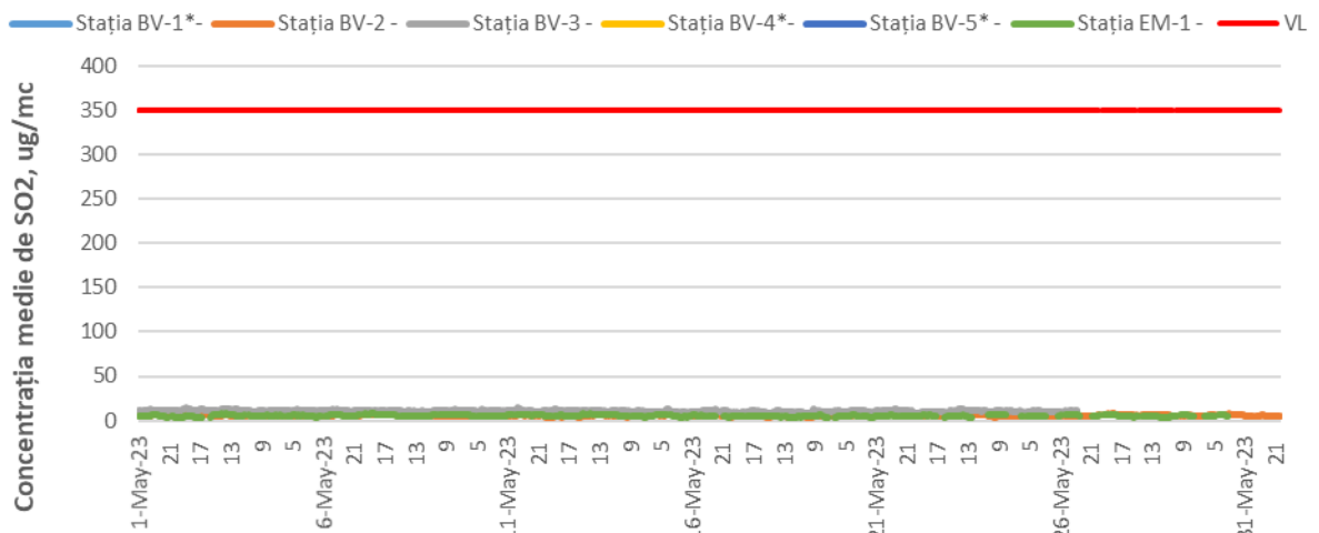
Figura 1.1.2.1.2. Evoluția mediilor orare de SO 2 în luna mai
